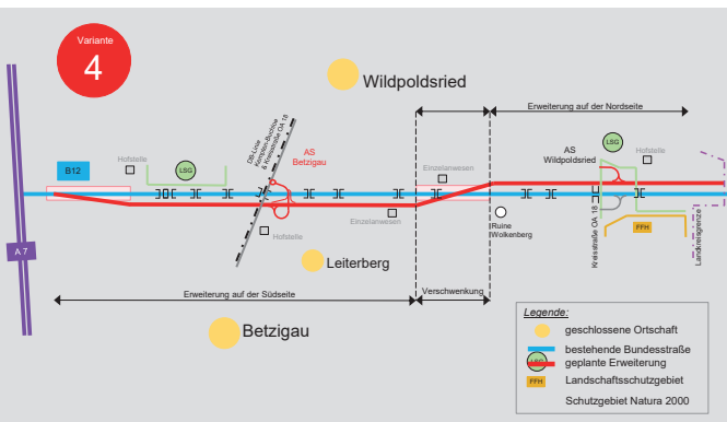
Planungsabschnitt 1 Kempten - Wildpoldsried Vorzugsvariante Süd Nord
